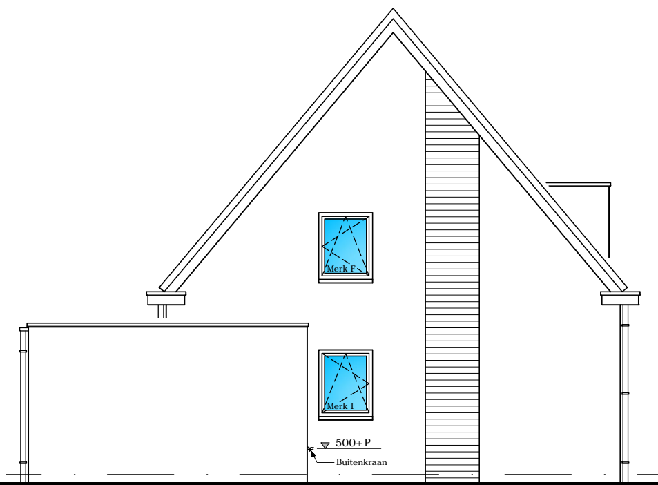
LINKER ZIJGEVEL
